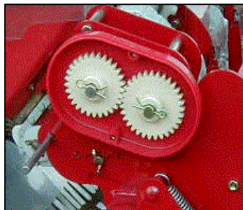
播種ピッチ変更部
