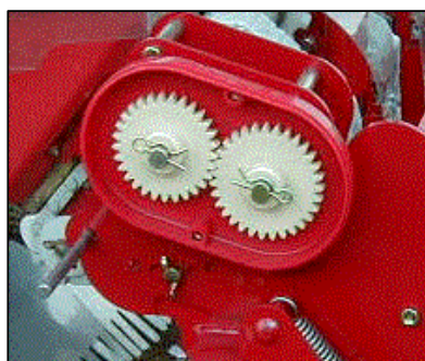
播種ピッチ変更部
