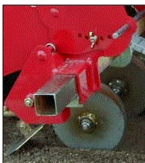
溝切り部ダブルディスク ベルト傾斜角度調節付き
