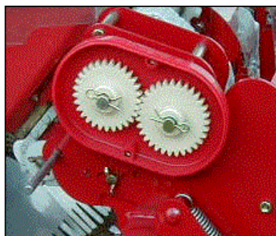
播種ピッチ変更部
